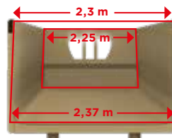
Conische laadbak (2,25 m vooraan en 2,3 m achteraan), breder onderaan dan bovenaan om het lossen te vergemakkelijken.
